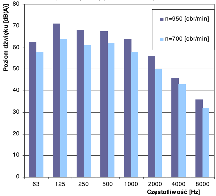
Poziomy dźwięku wentylatora WDC/s 50 z podstawą tłumiącą.
