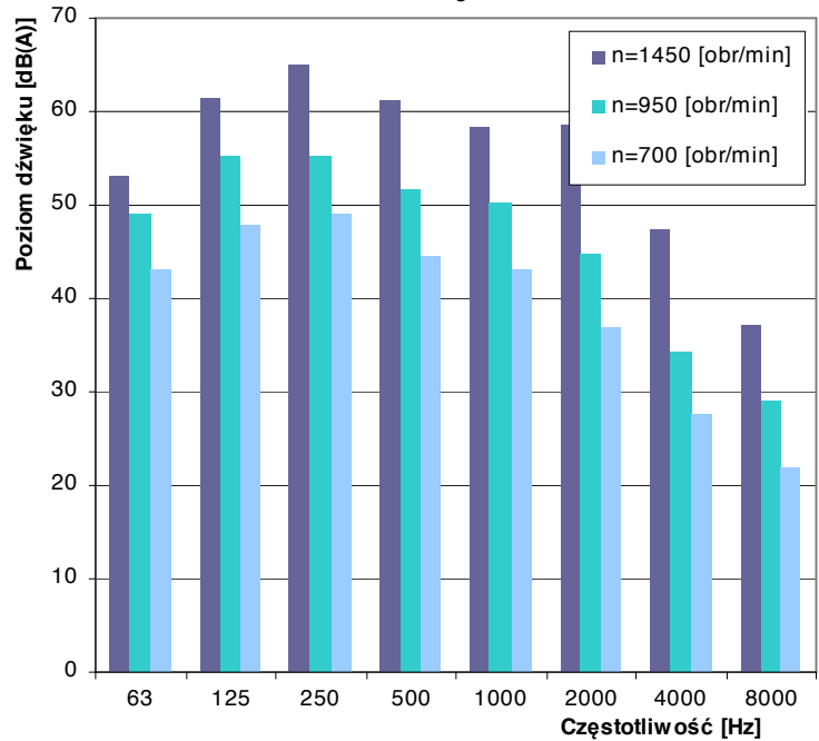
Poziomy dźwięku wentylatora WDC/s 20 dla poszczególnych częstotliwości
