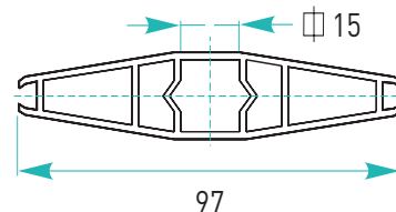
Rysunek 2. Lamela przepustnicy PWIIS.
