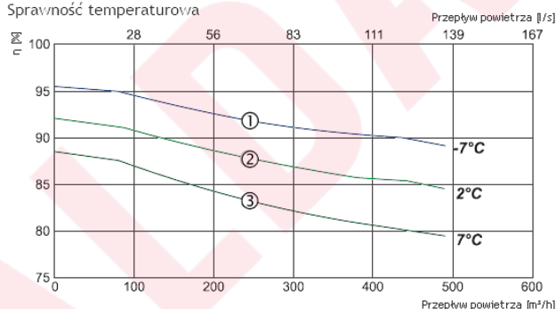
Sprawność temperaturowa
